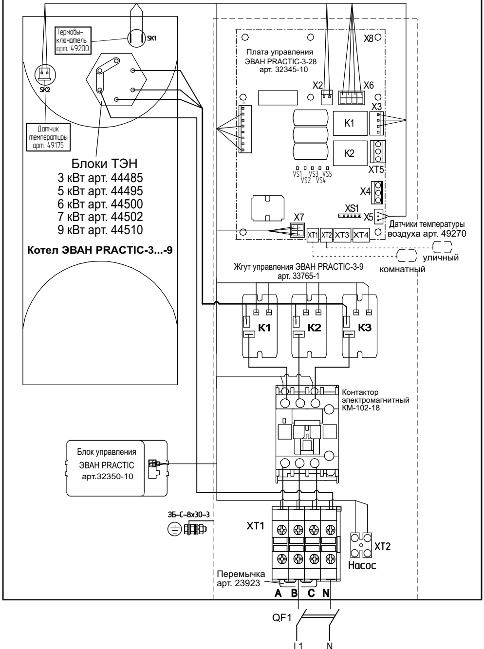
Рисунок 18. Схема подключения ЭВАН PRACTIC-3...-9 к сети 220В.
