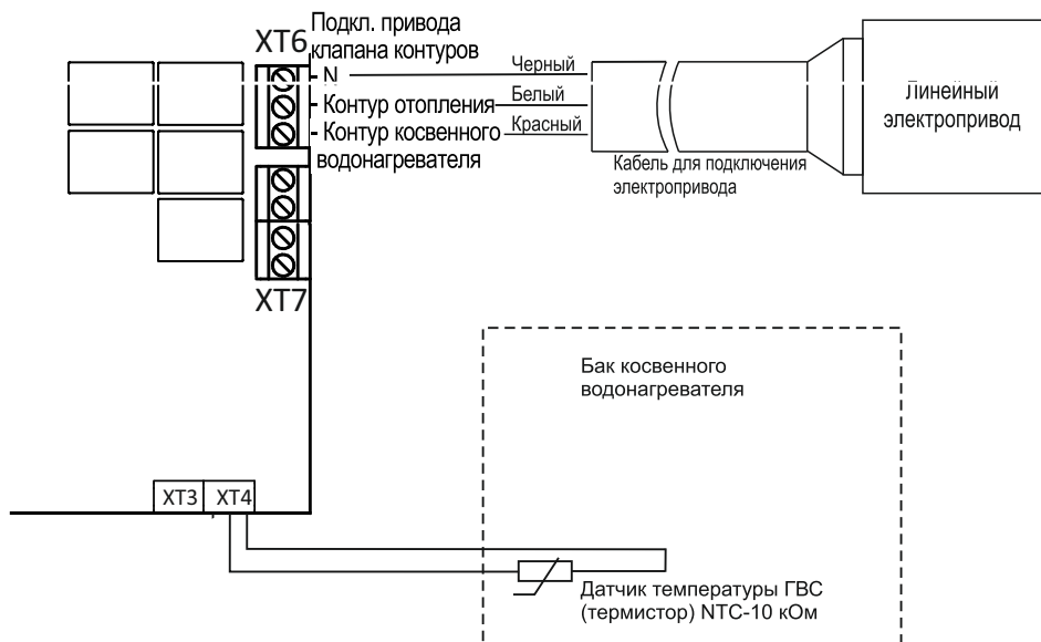
Рисунок 24. Электрическое подключение комплекта ГВС EVAN AQUA.
