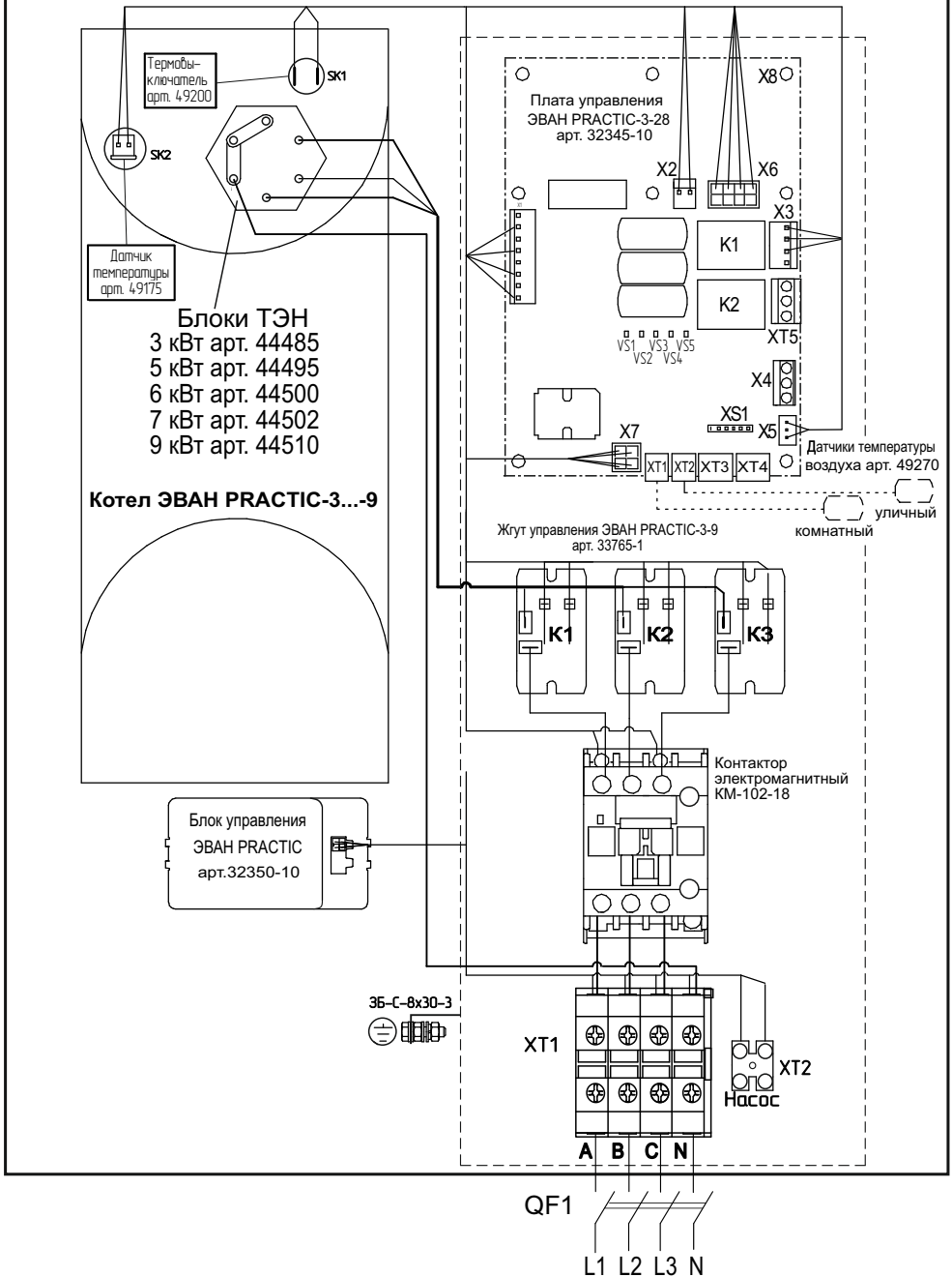
Рисунок 19. Схема подключения ЭВАН PRACTIC-3...-9 к сети 380В.
