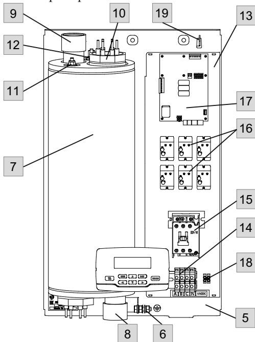
Рисунок 3. Прибор ЭВАН PRACTIC - 18 ... -28 со снятым кожухом.
