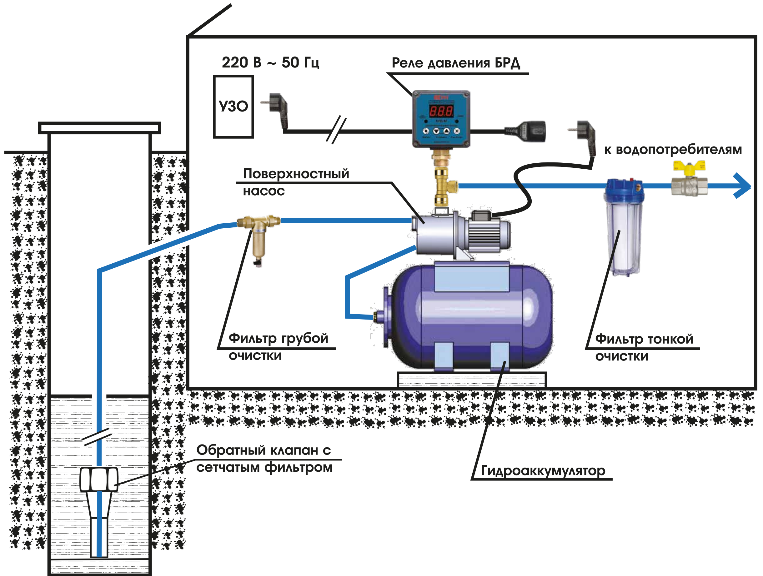
Схема 1. Подключение реле давления БРД "Акваконтроль" с поверхностным насосом
