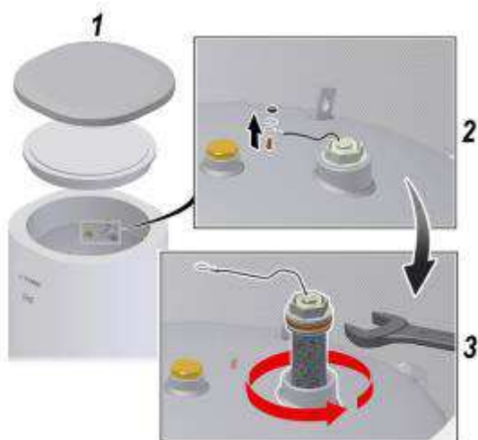
Рис. 10 Замена защитного магниевого анода
