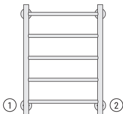
Нижнее подключение (в стену) для моделей Версия-Н1, Версия-Н2
