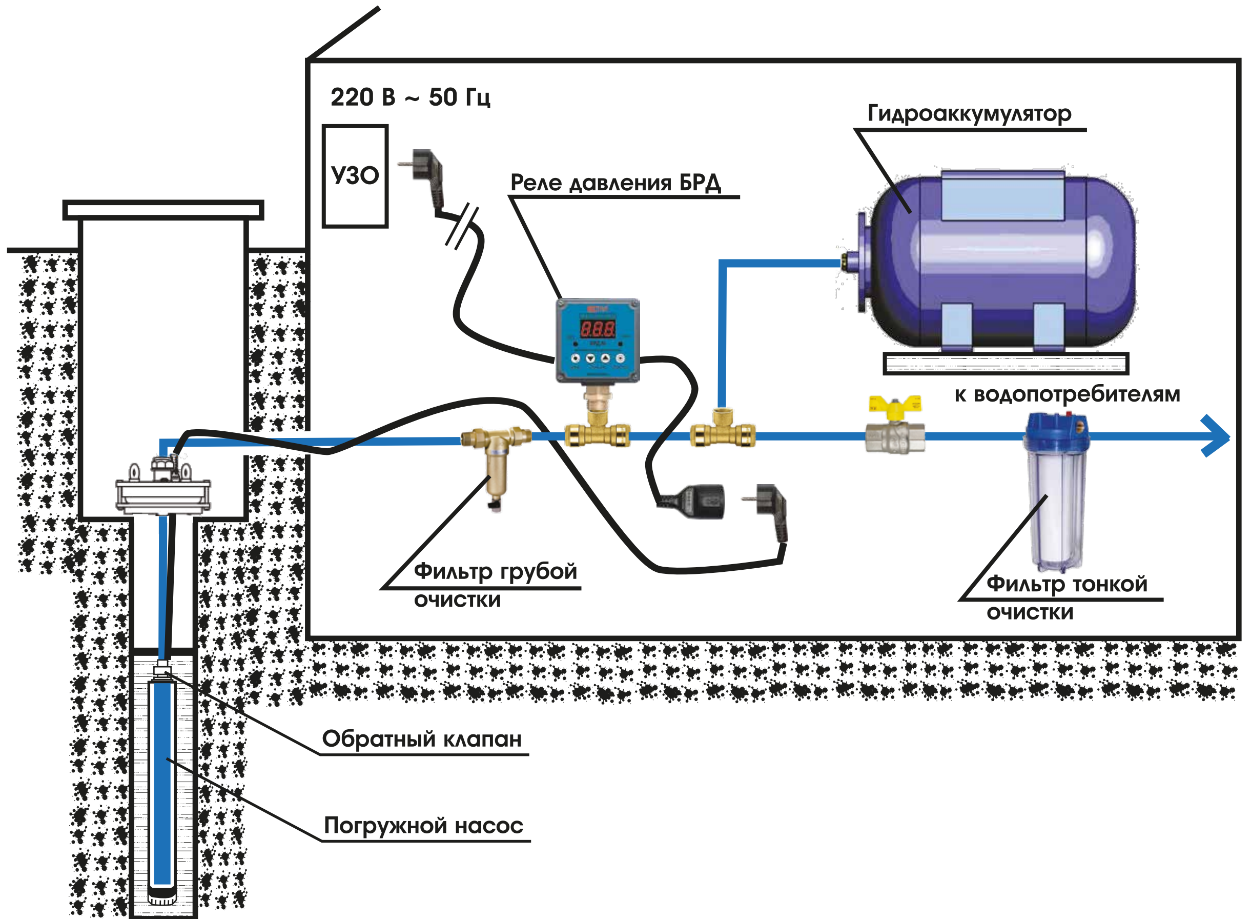
Схема 2. Подключение реле давления БРД "Акваконтроль" с погружным насосом
