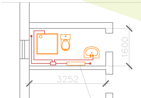
Горячее водоснабжение 2-го этажа
