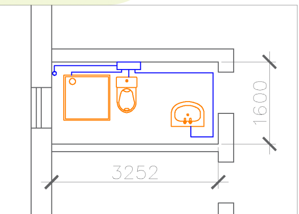
Водоснабжение 2-го этажа
