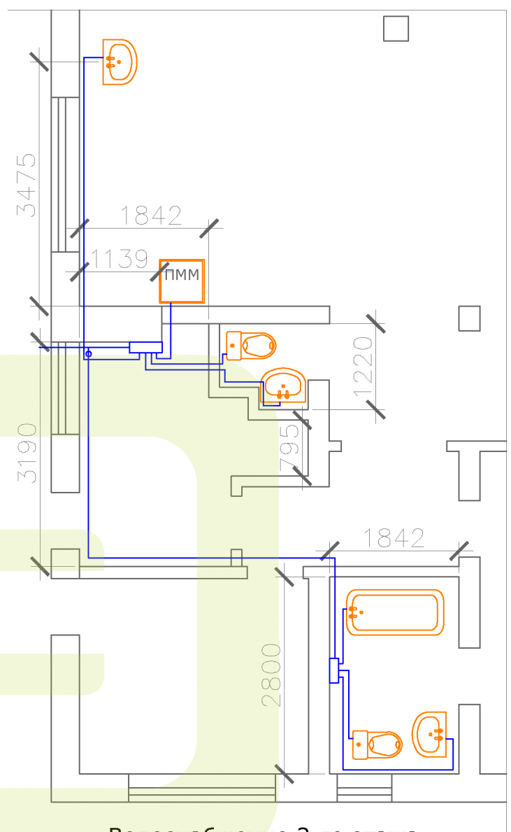
Водоснабжение 2-го этажа
