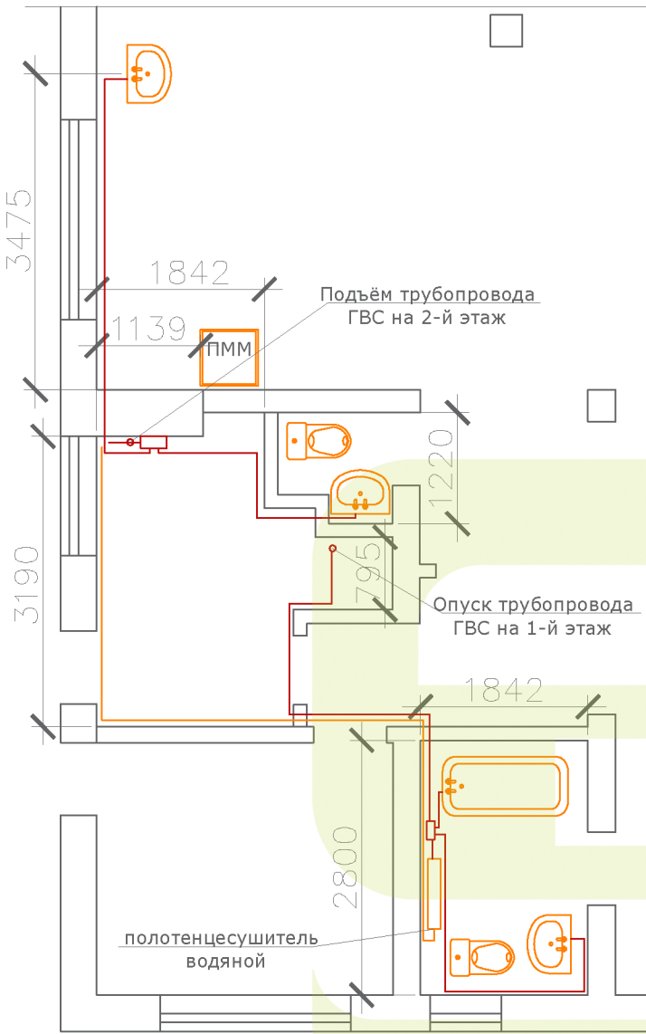
Горячее водоснабжение 2-го этажа
